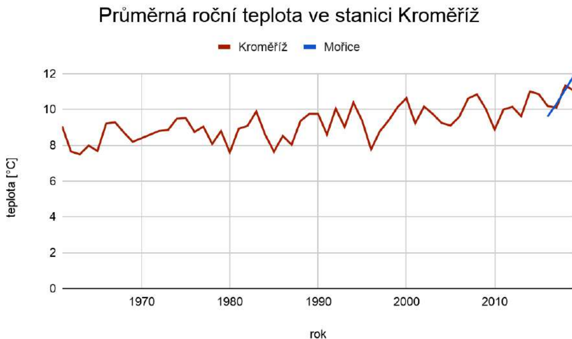
Obr. 38: Průměrná roční teplota (ve stanici Kroměříž)
